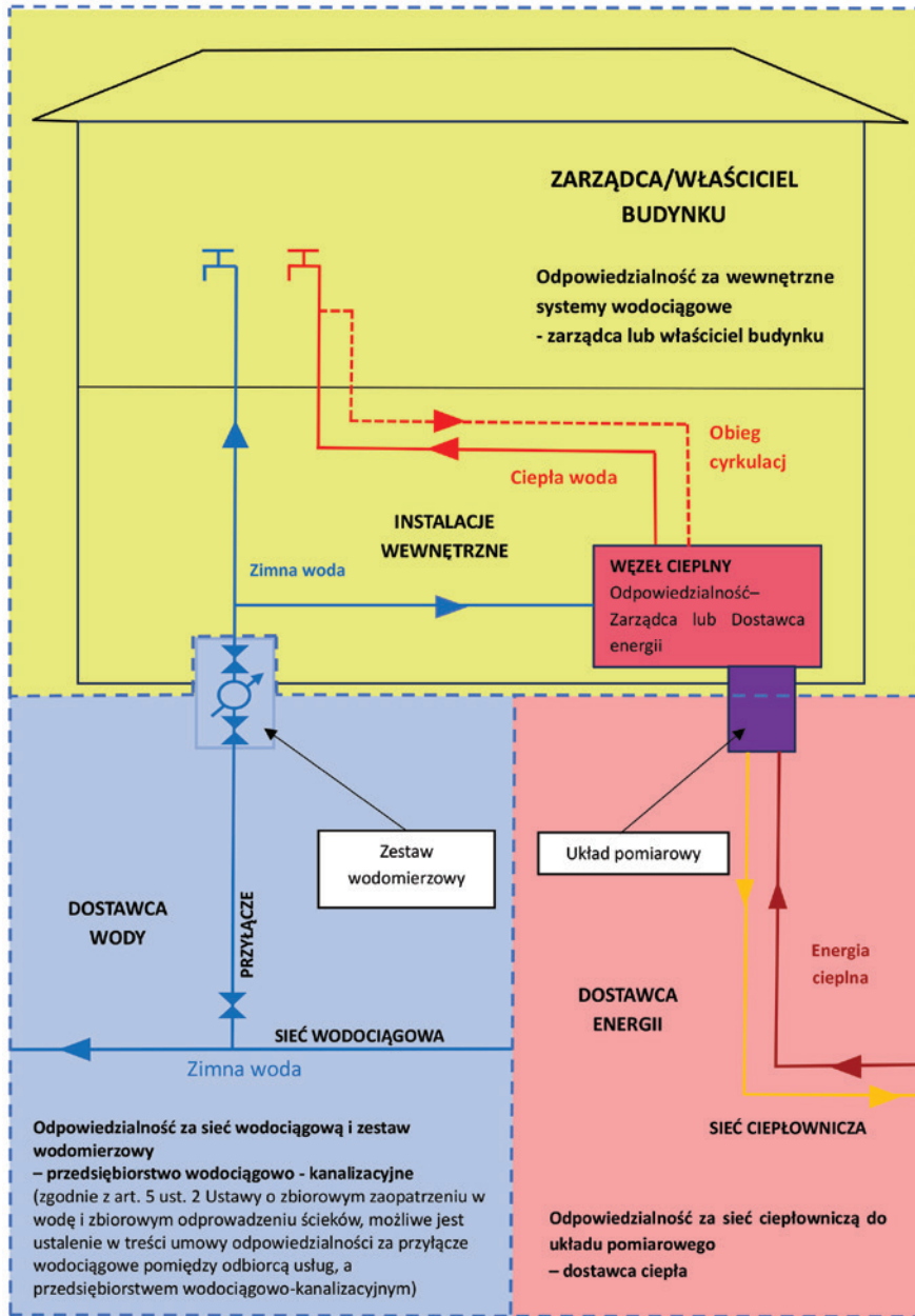
Rysunek 3. Podział odpowiedzialności za sieć/przyłącze/zestaw wodomierzowy/wewnętrzny system wodociągowy wody ciepłej i zimnej w budynkach wielolokalowych i innych wyposażonych w system cyrkulacji wody ciepłej.
