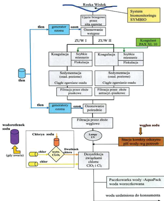
Rysunek 4. Uproszczony schemat technologiczny procesu uzdatniania wody w ZUW Zwiężczyca, woda surowa ujmowana jest z rzeki Wisłok
